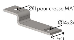
Type 3 : Z - H Oblong horizontal
