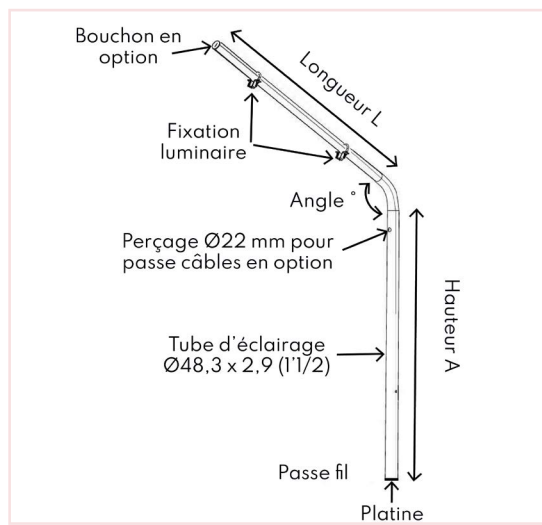
Etrier luminaire
